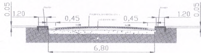
PERFIL TRANSVERSAL - RUA SDO 01
