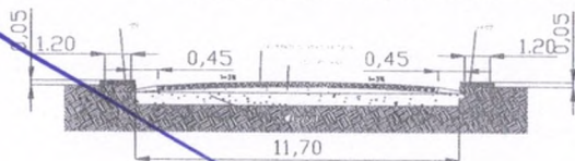
PERFIL TRANSVERSAL AVENIDA PREFEITO WILSON SAMPAIO
