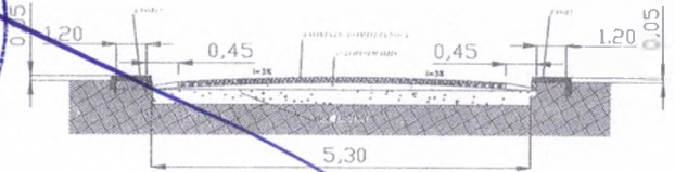
PERFIL TRANSVERSAL RUA ORLEANS FARIAS
