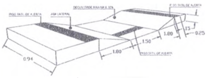
PERSPECTIVA DA RAMPA DE ACESSO
