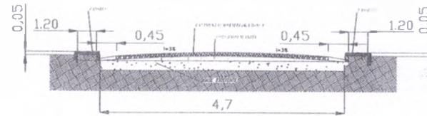
PERFIL TRANSVERSAL 2- RUA QUATRO
