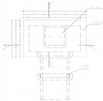
01 PLANTA BAIXA 0,40x0,40m
