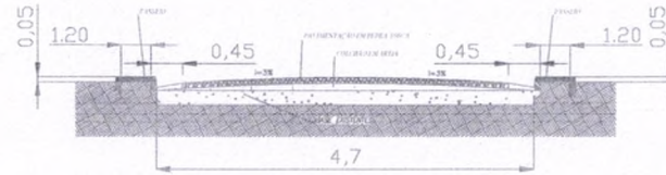
PERFIL TRANSVERSAL 2- RUA QUATRO
