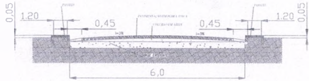
PERFIL TRANSVERSAL 1- RUA QUATRO
