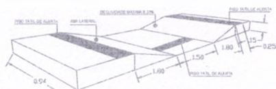
PERSPECTIVA DA RAMPA DE ACESSO
