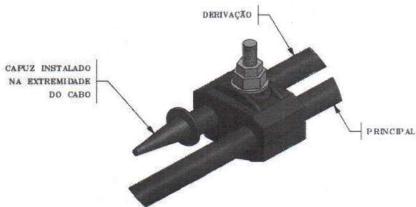
VISTA PERSPECTIVA MONTADO
