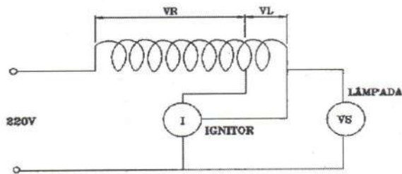
DETALHE 2
