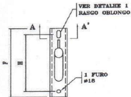
BASE DO BRAÇO VISTA FRONTAL
