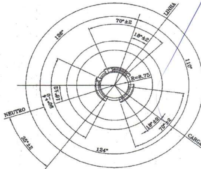
VISTA INFERIOR
