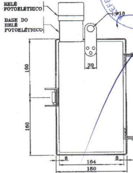
VISTA POSTERIOR
