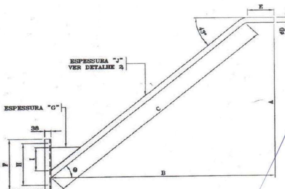
VISTA LATERAL
