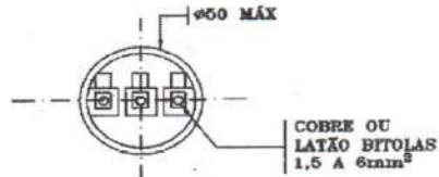
VISTA INFERIOR
