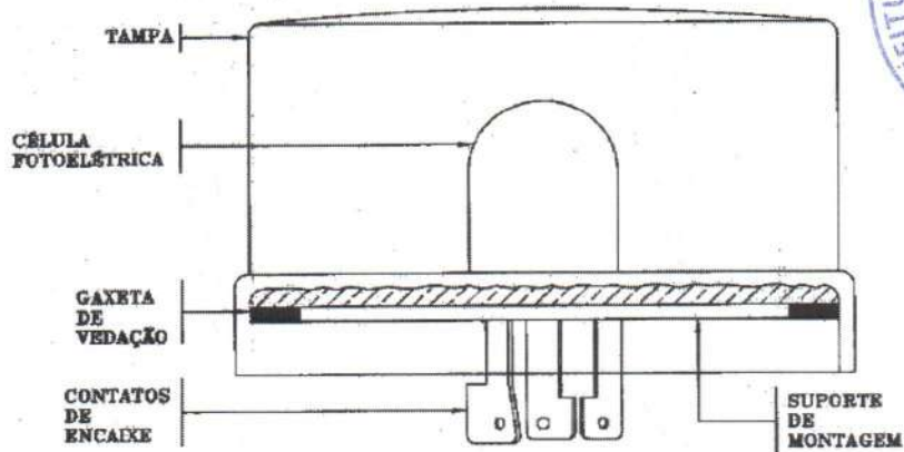
VISTA LATERAL
