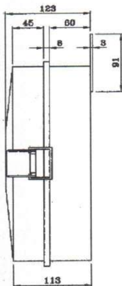
VISTA LATERAL ESQUERDA SEM RELÉ FOTOELÉTRICO E SEM A BASE DO RELÉ
