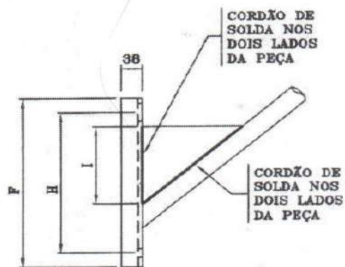
BASE DO BRAÇO VISTA LATERAL
