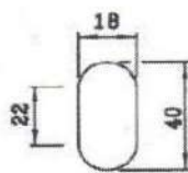
DETALHE 1 RASGO OBLONGO
